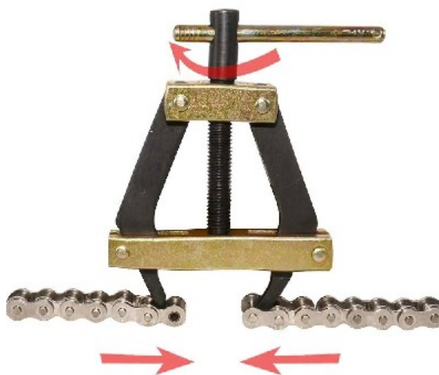
ALAT ZA SPAJANJE/STEZANJE LANCA
